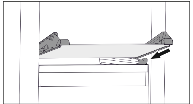
Fig. 108 Glasplatte des abklippbaren Schubfachs
