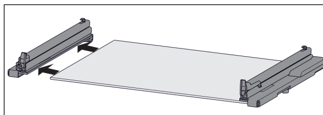
Fig. 98 Glasplatte mit Schienen
