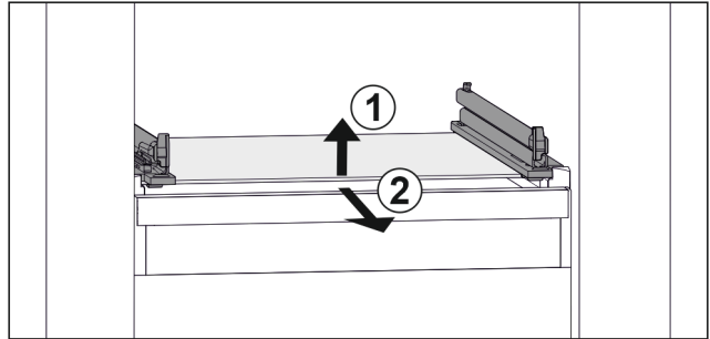
Fig. 87 Beispielhafte Darstellung der Glasplatte
